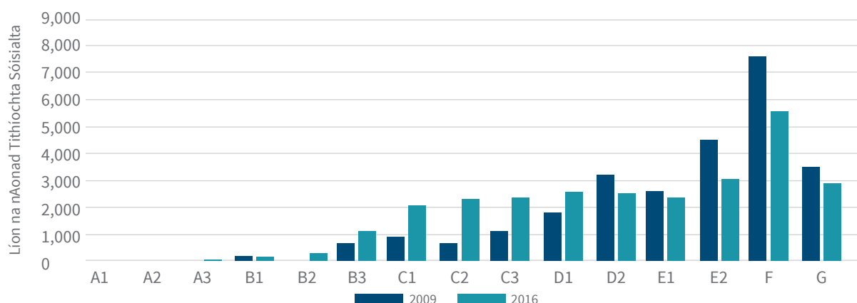
Fíor 24 Rátálacha Fuinnimh Foirgnimh do Stoc Tithíochta Sóisialta Chathair Bhaile Átha Cliath go léir in 2016
