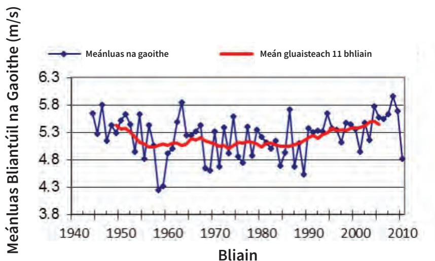
Fíor 7 Treochtaí Gaoithe Aerfort Bhaile Átha Cliath (1944-2010) (Foinse: An GCC / Dwyer)
