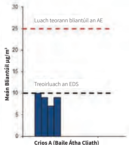
Fíor 16 Meándlúsanna Ábhair Cháithnínigh Bhlantúil PM_{2.5} (Mínábhair Cáithnínach) ag Stáisiúin Aonair in 2016 (Foinse: an GCC)
