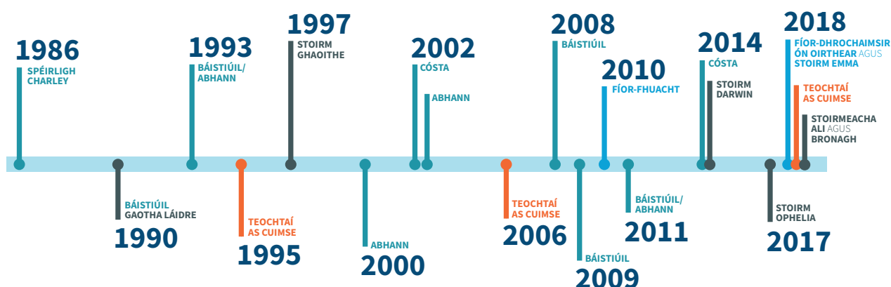
Fíor 4 Amhlíne na dTeagmhais Mór Aeráide i mBaile Átha Cliath
