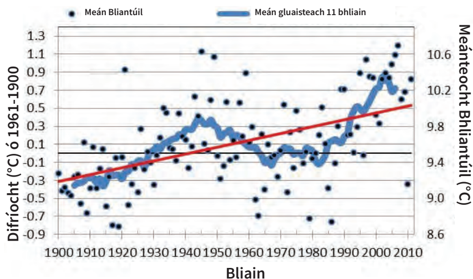
Fíor 6 Meánteocht Air Dromchla (1900-2011) (Foinse: An GCC / Dwyer)
