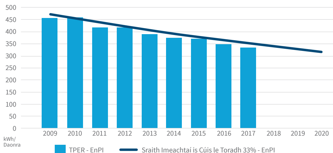
Fíor 22 Feidhmíocht Fuinnimh Bhliantúil CCBÁC i gComparáid leis an tSraith Imeachtaí is Cúis le Toradh 33%
