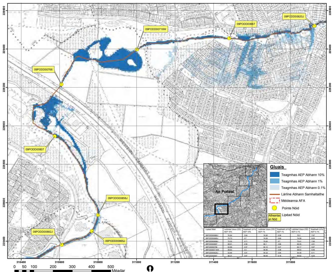
Fíor 9 Méideanna Tuile Abhann Bhaile Átha Cliath Theas (Foinse: Anna Oiriúnú ón Taifead ar Dhéanmhais Chosanta/Oifig na nOibreacha Poiblí)
