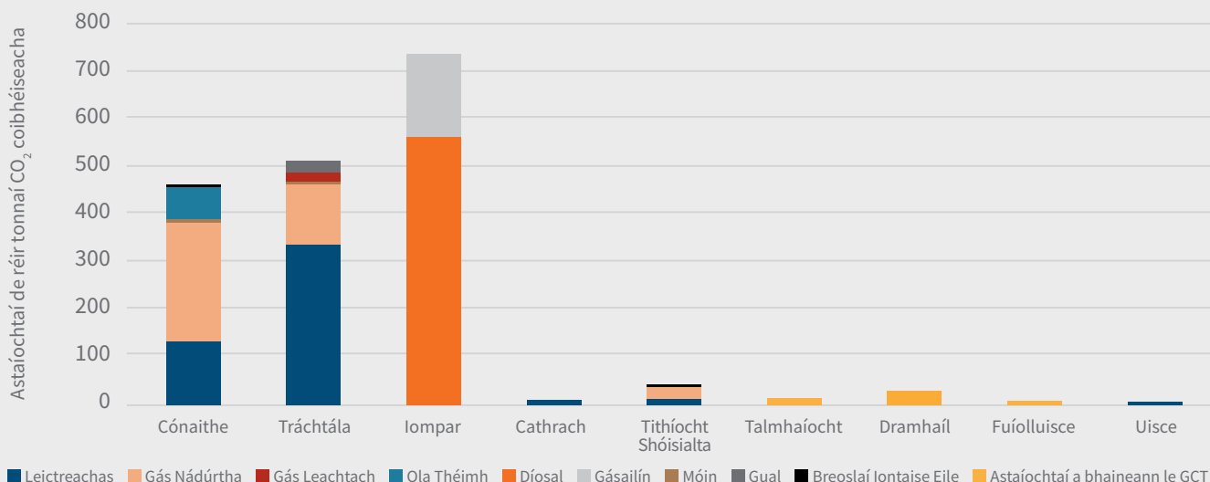
Fíor 22 Astaíochtaí iomlána i dtonnaí dé-ocsáid charbóin coibhéiseacha in Earnálacha Éagsúla
