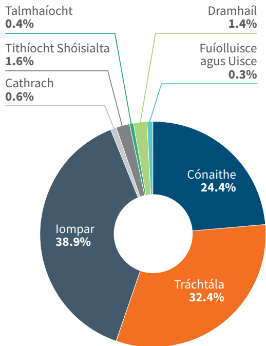
Fíor 19 Astaíochtaí Iomlána Gás Ceaptha Teasa do Bhaile Átha Cliath Theas in aghaidh na hEarnála
