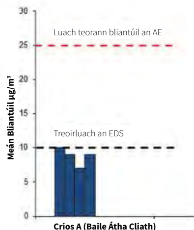
Fíor 10 Meándlúsanna Ábhair Cháithnínigh Bhliantúil 2.5 (Mínábhar Cáithnínach) ag Stáisiúin Aonair in 2016 (Foinse: an GCC)
