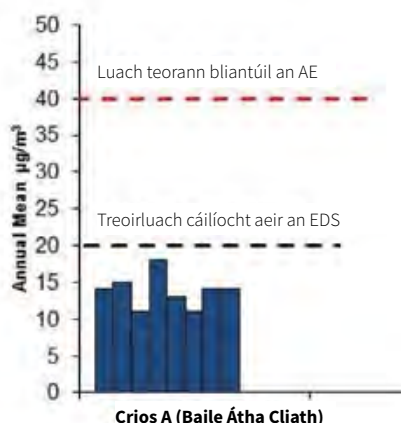
Fíor 11 Meándlúsanna Ábhair Cháithnínigh Bhliantúil 2.5 ag Stáisiúin Aonair in 2016 (Foinse: an GCC)
